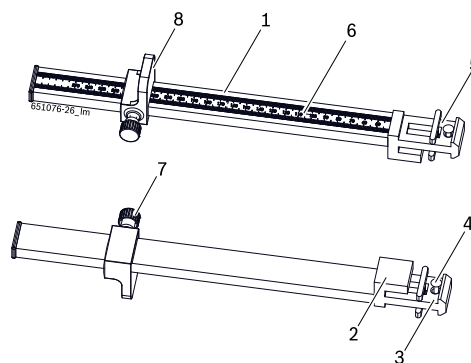
Fig. 36: Калибр позиционирования грузов
