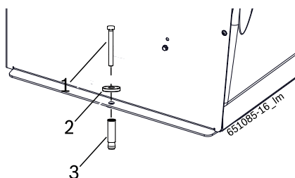
Fig. 17: Фиксация SBM V660 A
