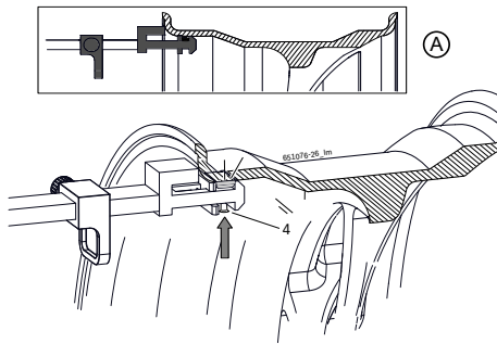
Fig. 37: Пример применения внутреннего адгезивного груза
