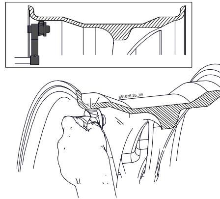
Fig. 34: Пример применения внутреннего адгезивного груза
