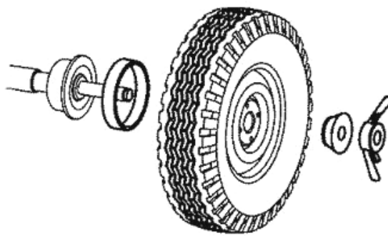
г - конус \varnothing 97 \dots 160 с кольцом
